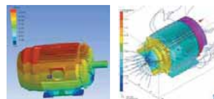
Анализ распределения механической и тепловой нагрузки
